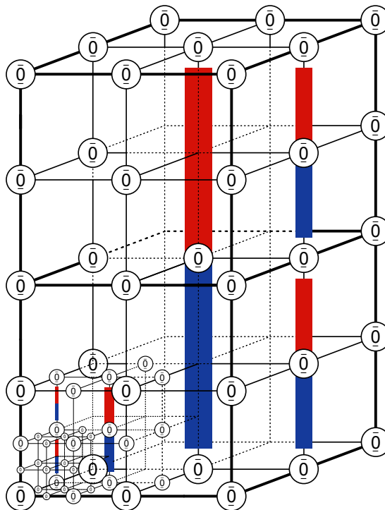
Abb. 26 Polarität in kubischen Wellenfeldern
