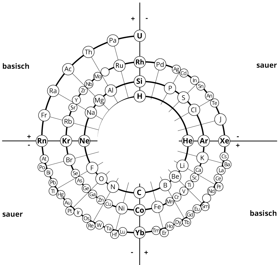
Abb. 9 Das Periodensystem der Elemente in Spiralfarm mit ergänzten Unterteilungslinien
