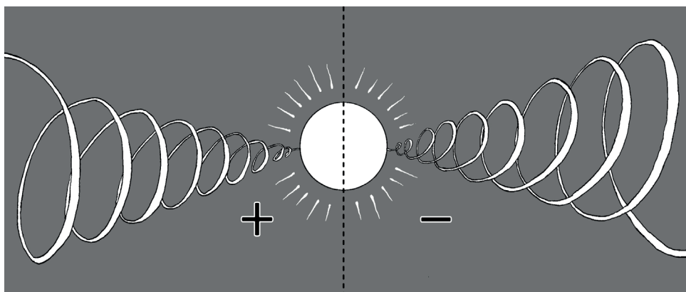
Abb. 28 Detailansicht um die Kugelbildung: Rechtsdrehende (+) und linksdrehende (-) Wirbel.
