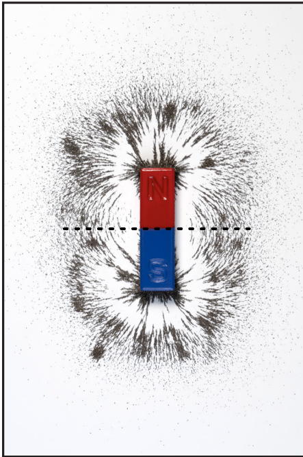
Abb. 22 (Oben links) Stabmagnet mit Magnetlinien
