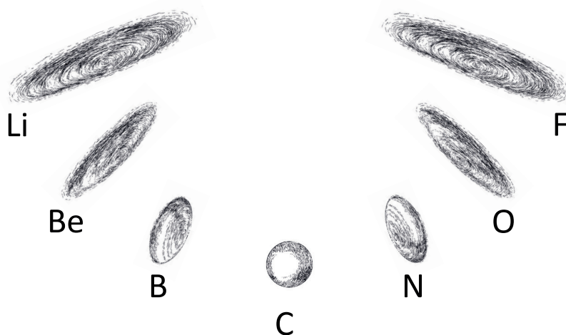
Abb. 39 Detailansicht der zweiten Oktave: Atomare Verdichtung und Entdichtung.
