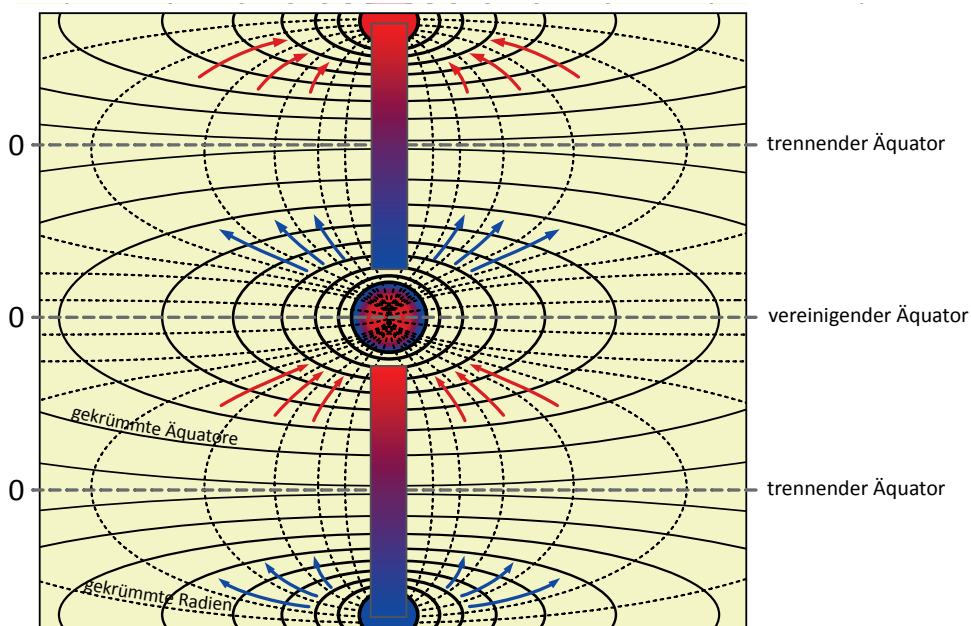
Abb. 27 Zwei Stabmagnete ungleicher Polarität bilden eine Kugel am vereinigenden Äquator.
