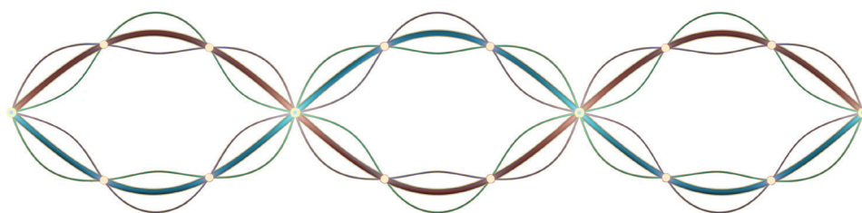
Abb. 36 Wirbelbewegung im Wellenfeld
