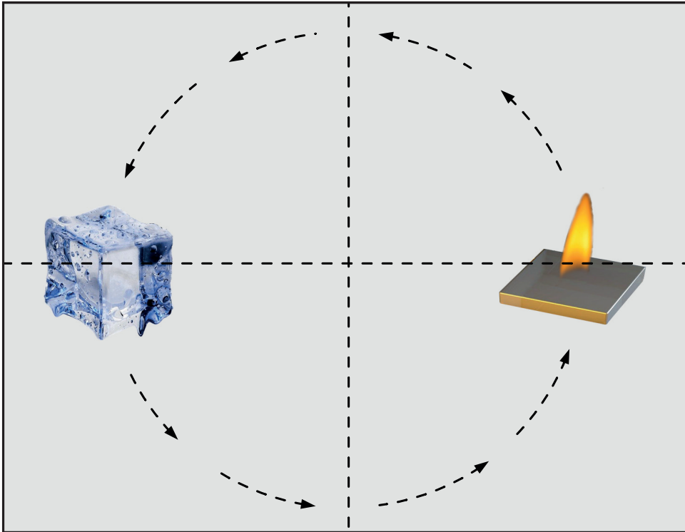
Abb. 25 Temperaturlausgleich durch Strömungsbewegung
