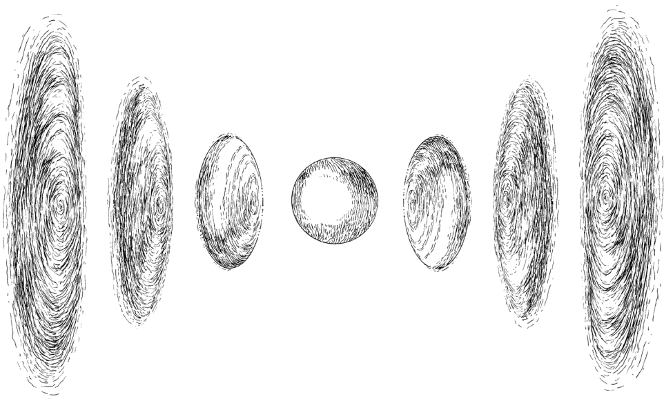
Abb. 35 Zyklisches Entstehen und Vergehen von Materie.
