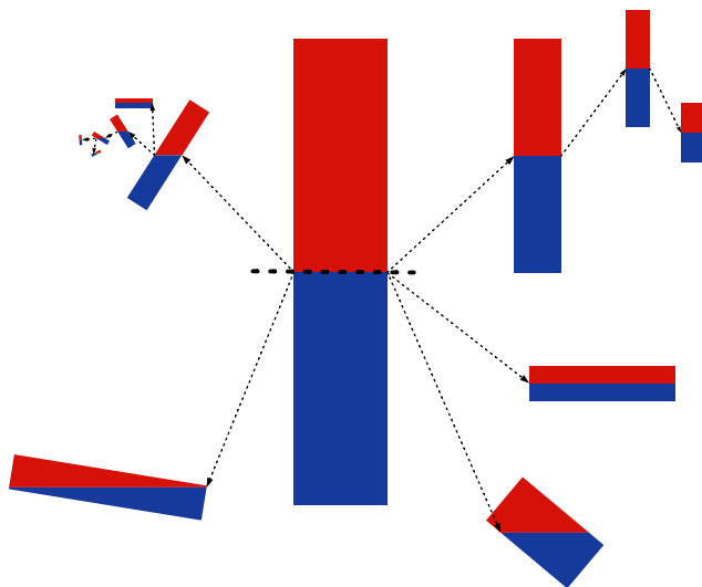
Abb. 24 (Rechts) Eisen, Kobalt und Nickel werden von einem starken Magneten mag- netisiert und damit selbst zu einem zweipoligen Magneten. Ihr Äquator ist am Äquator des Mag- neten ausgerichtet.
