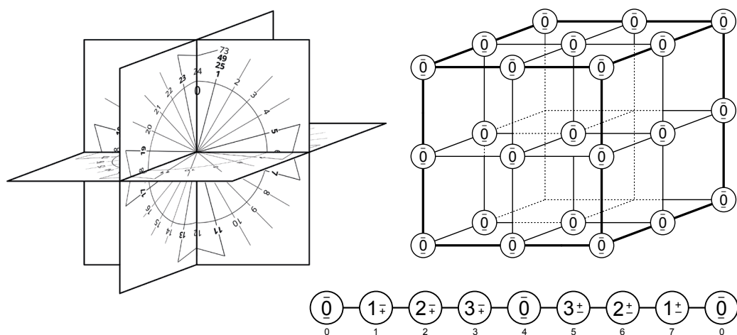
Abb. 32 Primzahlkreuz im Kubus sowie Position der Äquatoren in fortlaufenden kubischen Wellenfeldern.
