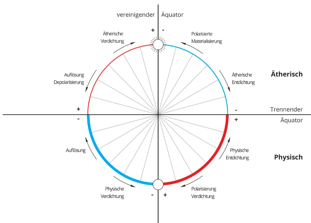
Abb. 21 Verdichtung und Entdichtung von Atomen
